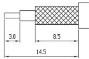
Recommend Cable Stripping Die Size A Die Size B
